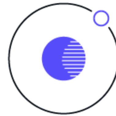
ATOMS
